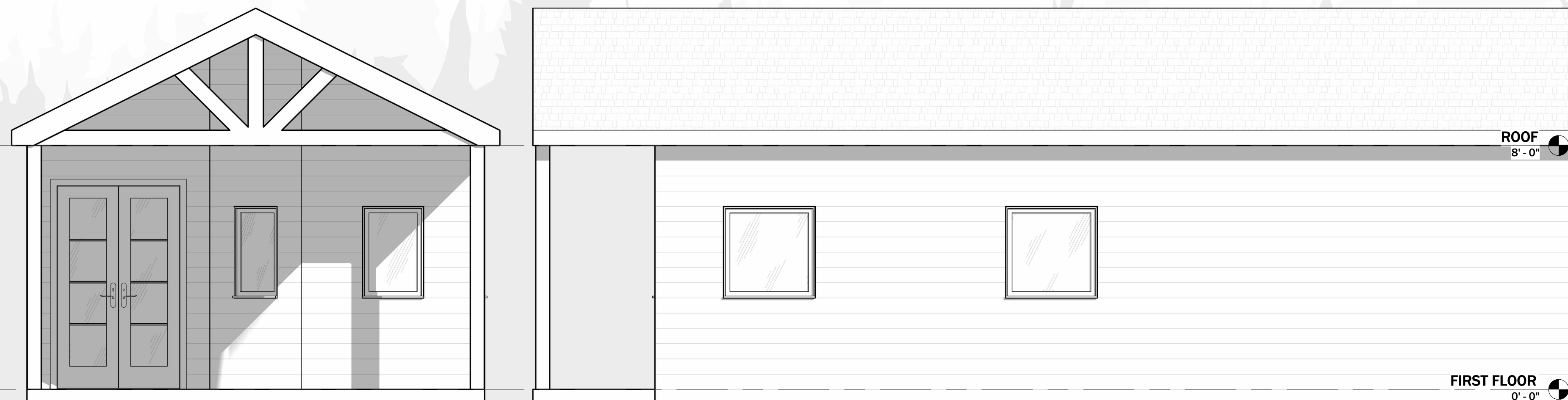
2 FRONT ELEVATION SCALE: 3/8" = 1'-0"
